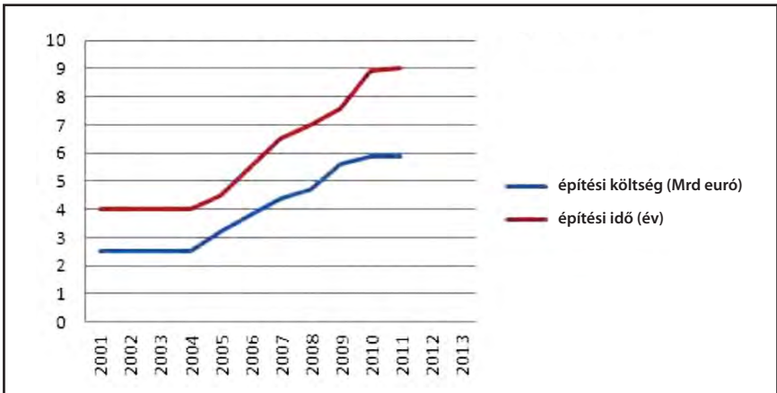
Finn nukleáris program (Olkiluoto): költségnövekedés
